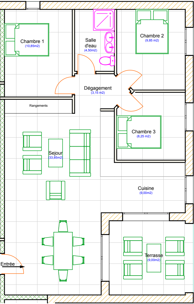
Appartement 8 1:100
