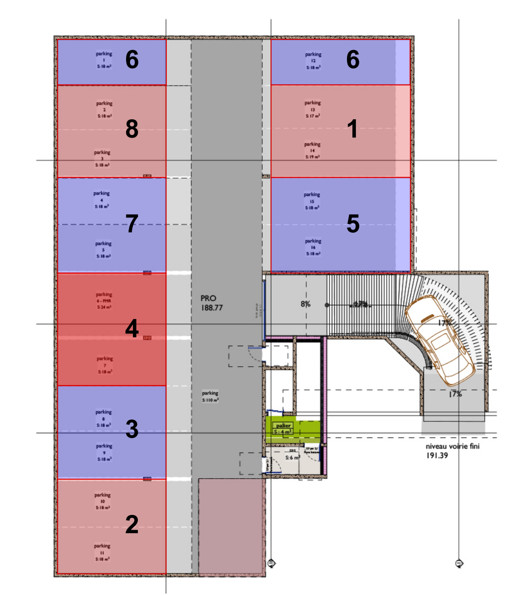
0. Parkings boxés + prise recharge véhicule 1:200
